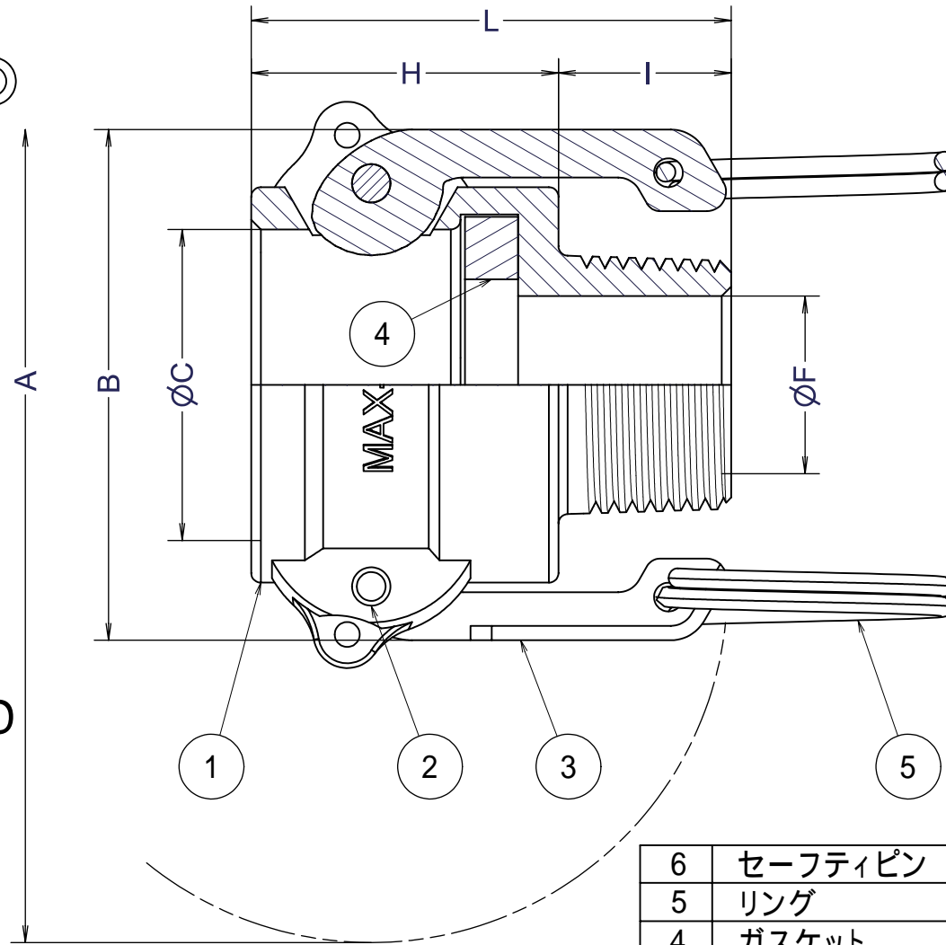
Section D-D
