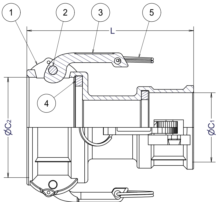
Section D-D
