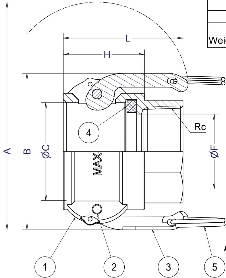
Section A-A
